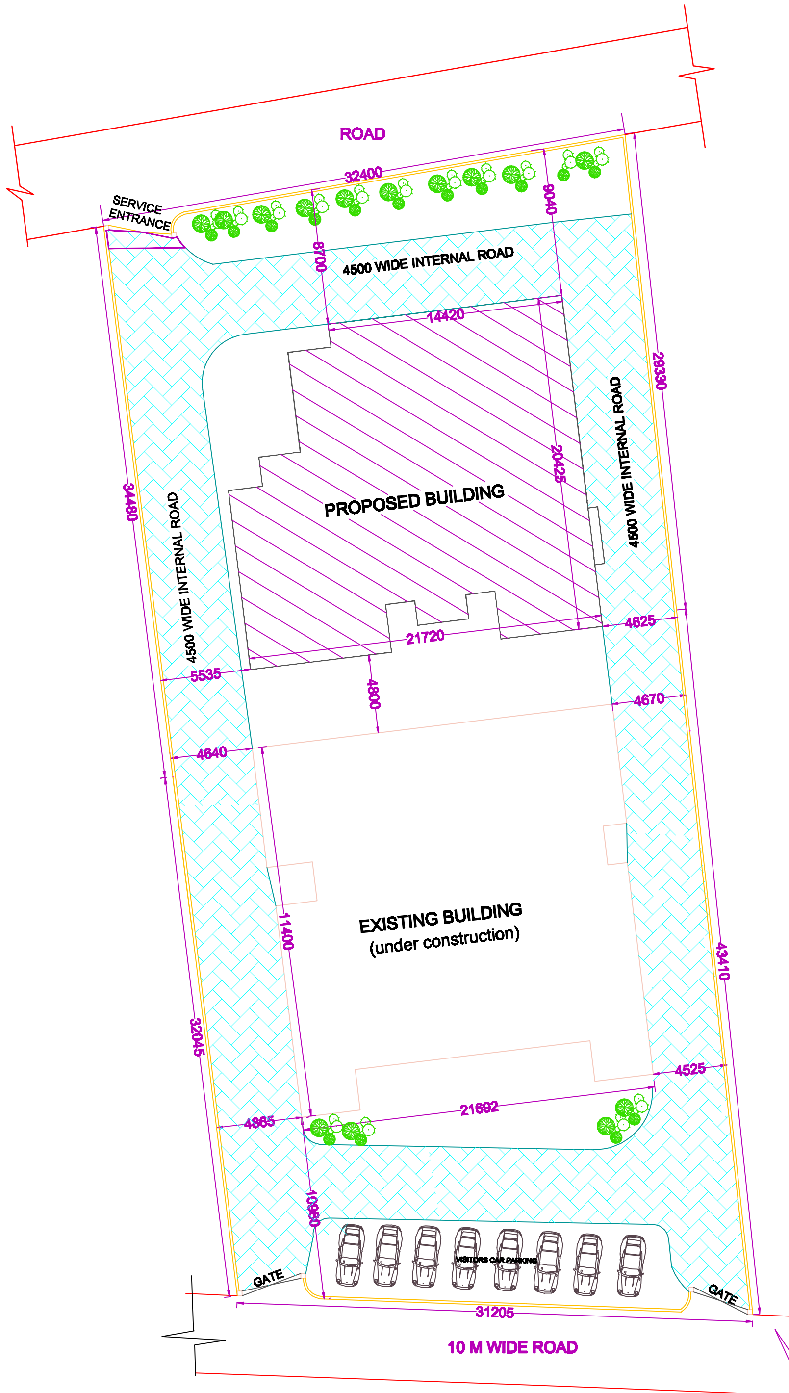
SITE PLAN N SCALE : 1:200
